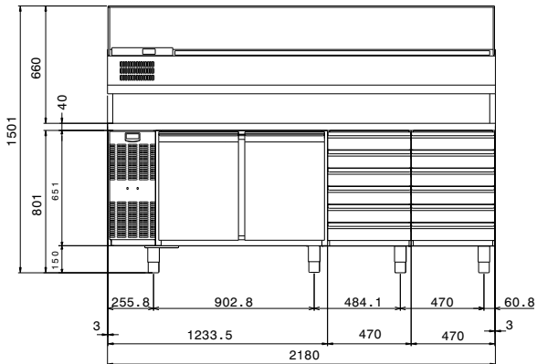
Front aanzicht
